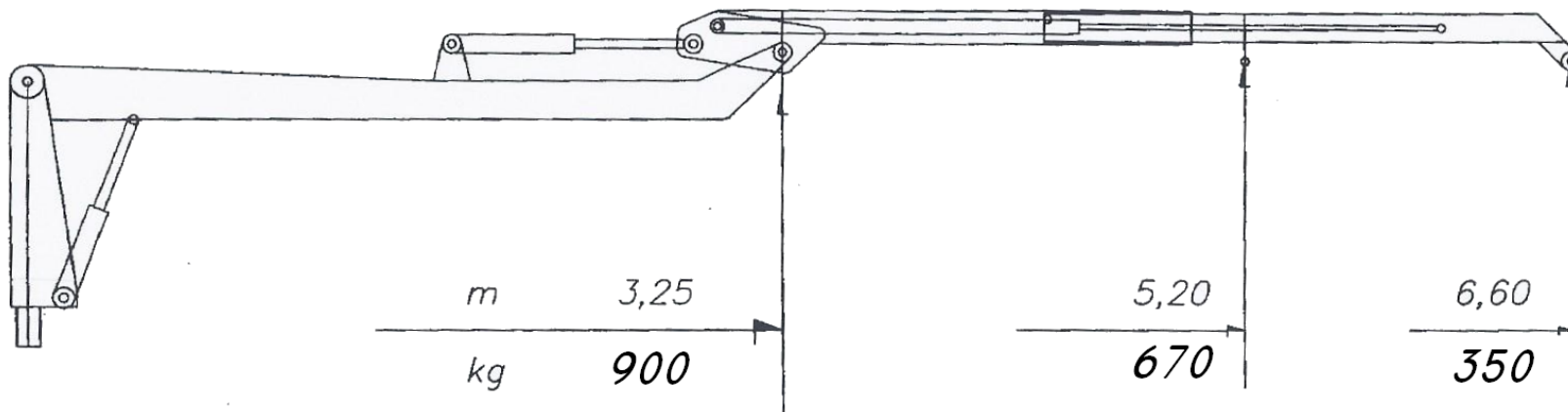
LASTDIAGRAMM DLUGPOL KRAN 660
